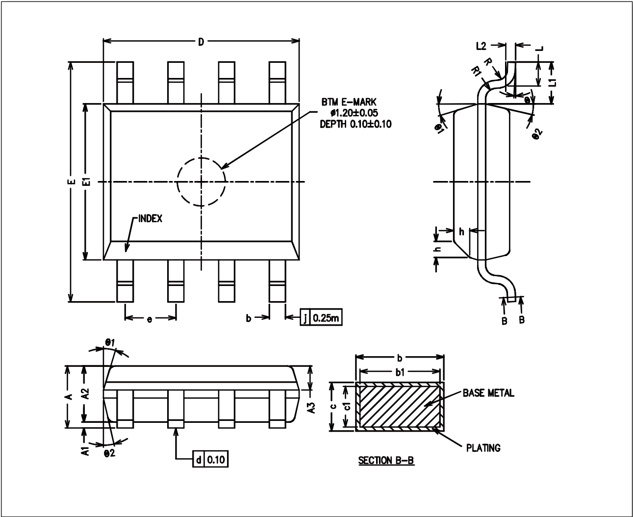
图 6-3 SOP8 封装尺寸
