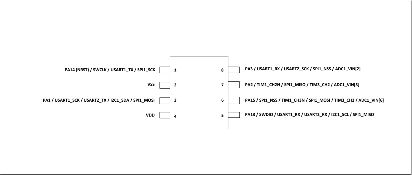
图 4-3 SOP8 – type 0 引脚分布
