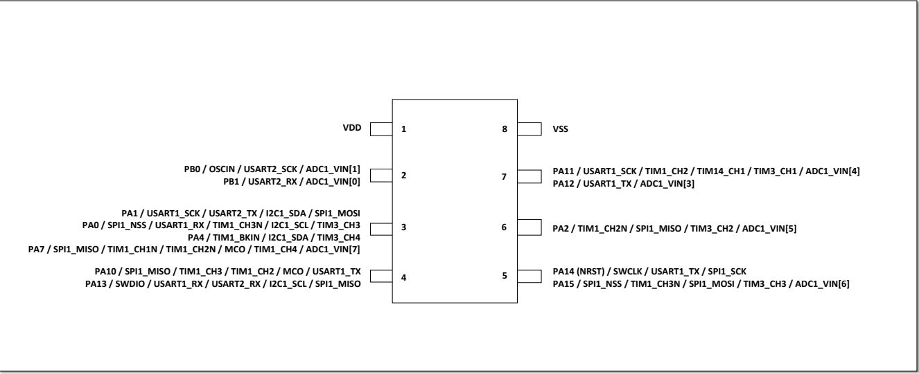
图 4-4 SOP8 – type 1 引脚分布
